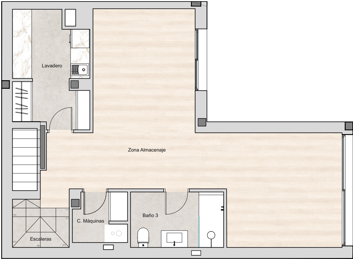
PLANTA SÓTANO
